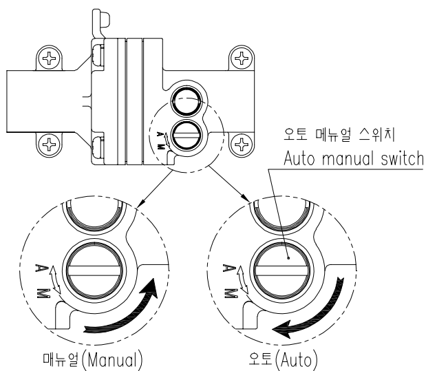
图7-13: A/M开关调节
