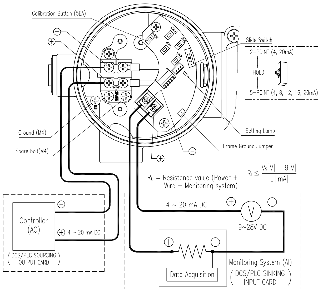
图6-5: 连接电缆
