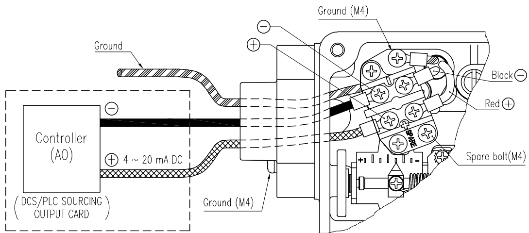
图6-4：连接电缆
