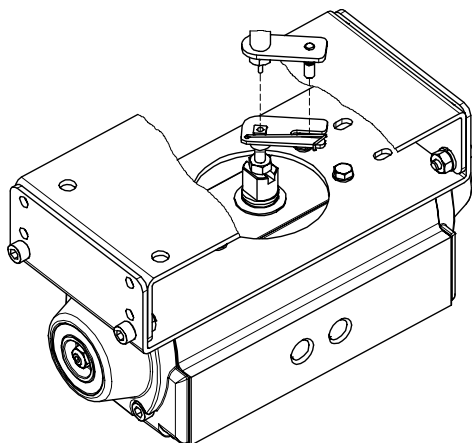
图4-17: 主轴中心对齐(叉杆)
