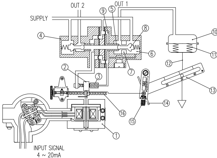
图3-1: 带执行器的直行程定位器
