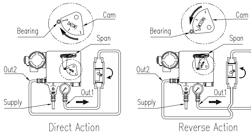
图5-9: 设置角行程双作用执行器的管路和凸轮的方向
