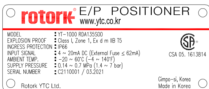
图L-6: YT-1000 I类, 1区, Ex d m IIB T5 (CSA) (-20 ~ 60 °C, NBR 橡胶)
