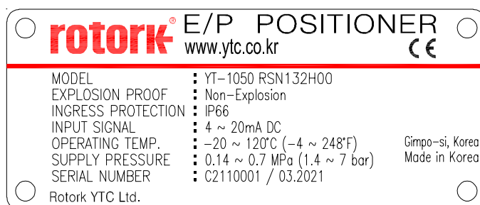
图L-21: YT-1050 非防爆型
