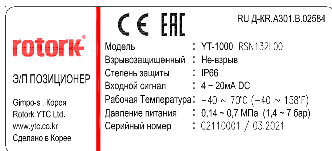
图L-2: YT-1000 非防爆型 (EAC)
