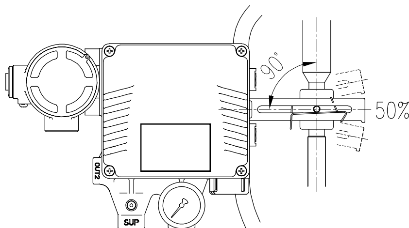
图4-7: 反馈杆和阀杆
