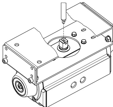
图4-18: 主轴中心对齐(Namur)
