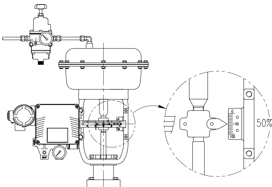
图4-5: 将阀门置于总行程50%的位置
