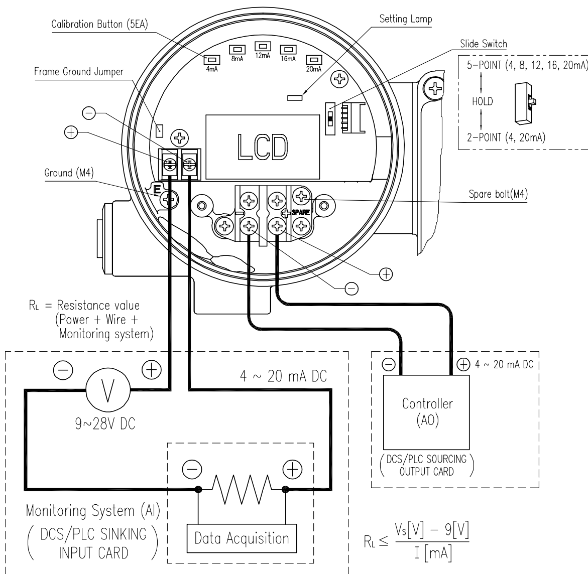
图6-6: 连接电缆
