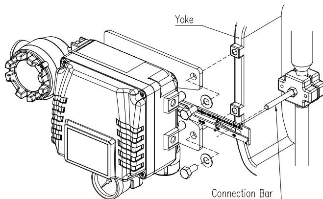
图4-4: 将支架安装于执行器轭上
