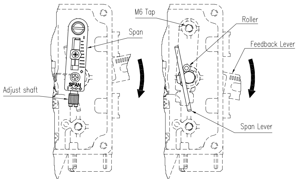
图7-1: 跨度件安装
