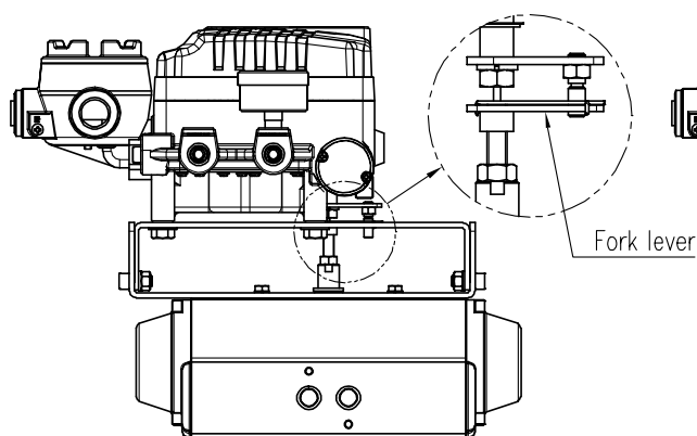
图4-10: 叉杆型
