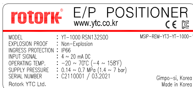
图L-1: YT-1000 非防爆型
