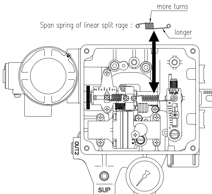
图7-17：直行程定位器
