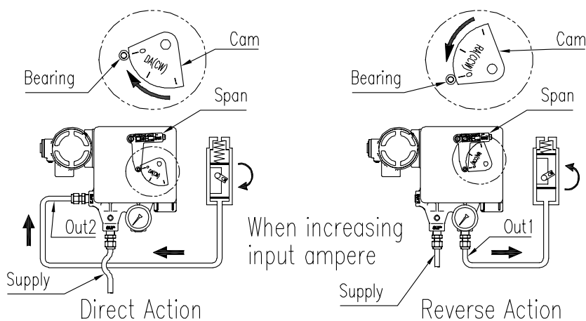
图5-5：设置角行程单作用执行器的管路和凸轮的方向
