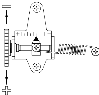
图7-8: 零点单元
