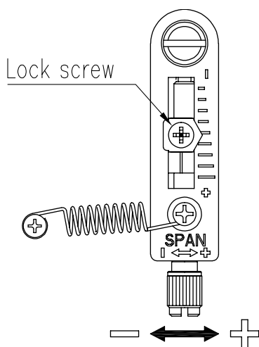
图7-9: 直行程跨度件单元
