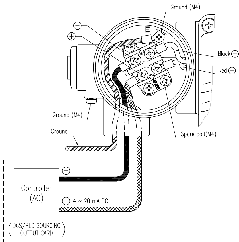
图6-3: 连接电缆
