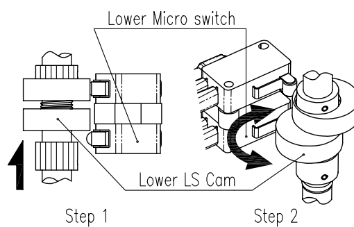
图7-12: 设置下部开关
