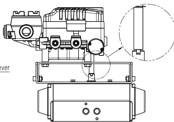
图4-11: Namur型
