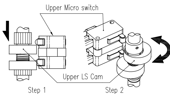
图7-11: 设置上部开关
