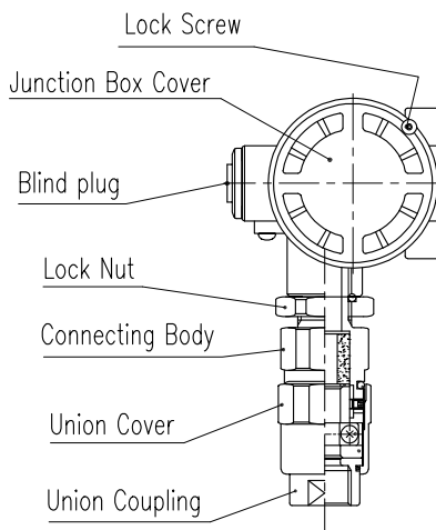
图6-1: 耐压填料管接头
