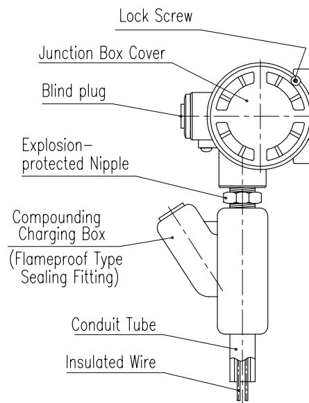
图6-2: 防火型复合加料箱
