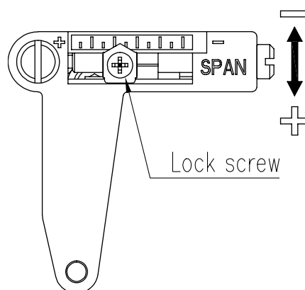
图7-10: 角行程跨度件单元
