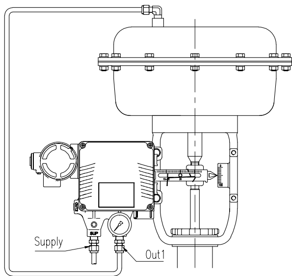
图5-1：单作用直行程执行器
