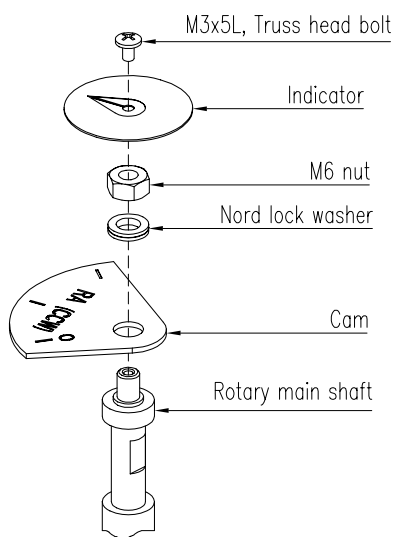
图7-6: 部件 (标准)
