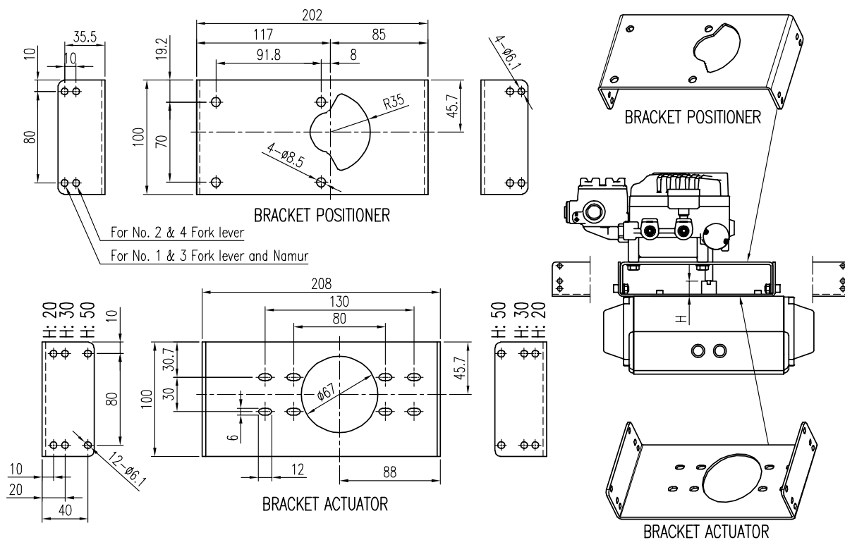
图4-12: 支架和定位器
