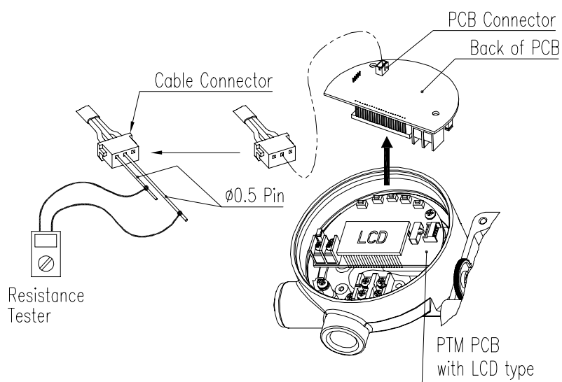
图7-16: 重置电位计电阻 (带LCD)
