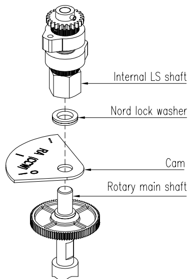
图7-7: 部件 (LS内部)
