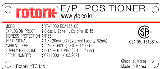
图L-7: YT-1000 I类, 1区, Ex d m IIB T5 (CSA) (-40 ~ 60 °C, 硅橡胶)
