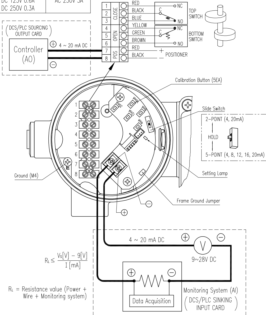
图6-7: 连接电缆
