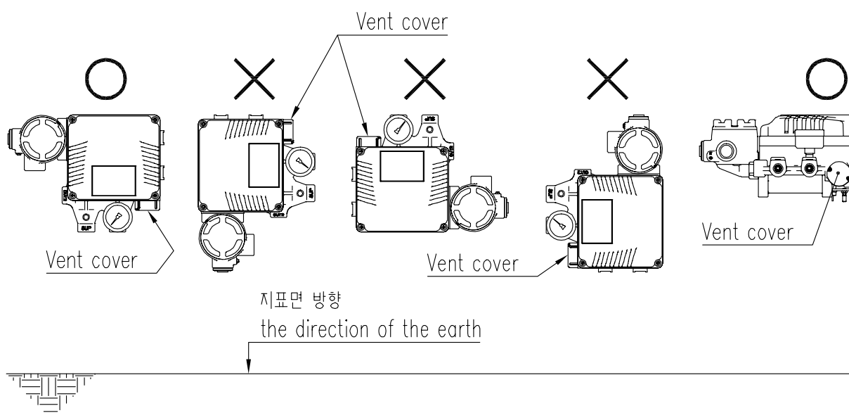
图4-1: 正确的通风盖位置
