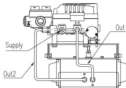
图5-7: 双作用角行程执行器
