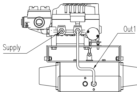
图5-2：单作用角行程执行器
