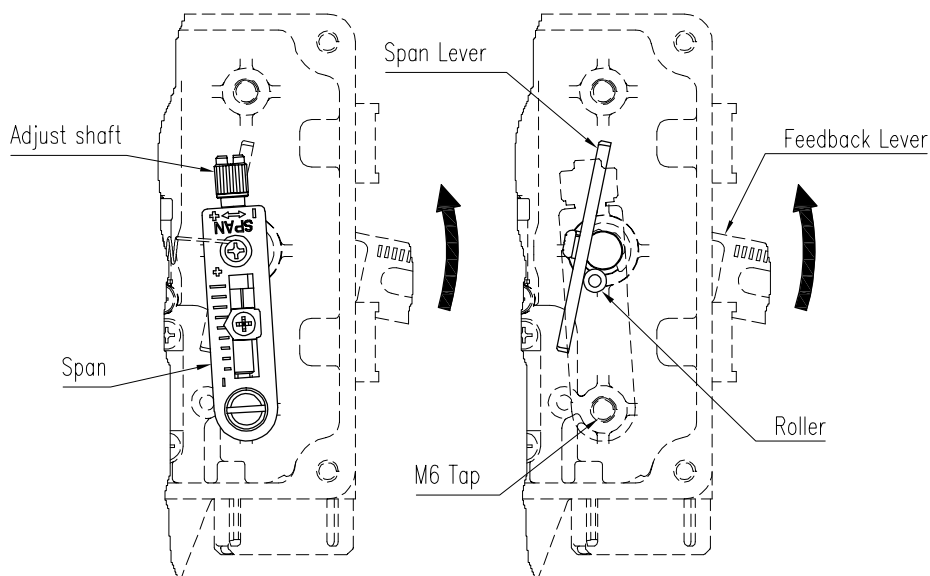
图7-3: 跨度件安装 (RA)
