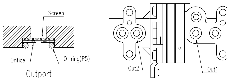
图7-14: 安装孔口件
