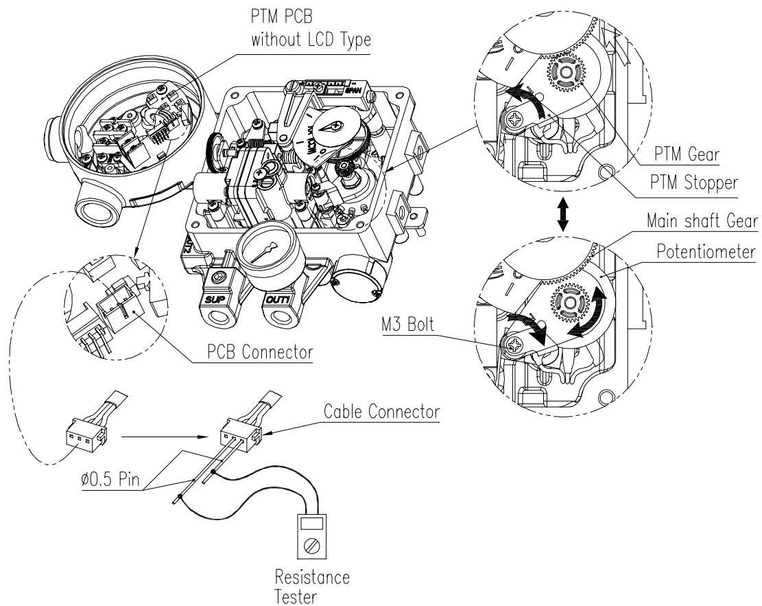
图7-15: 重置电位计电阻 (无LCD)
