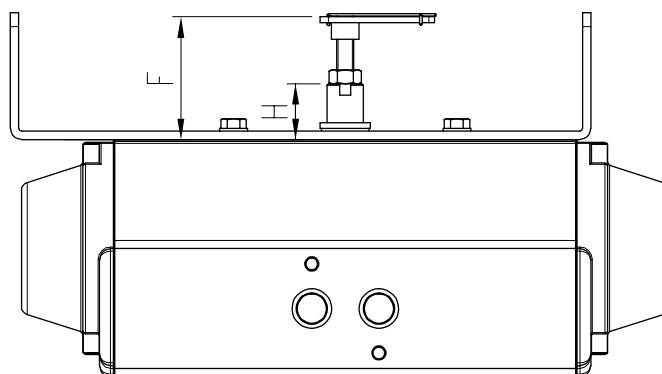
图4-16: 叉杆高度
