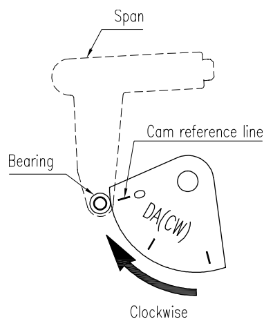
图7-4: 凸轮安装 (Da)
