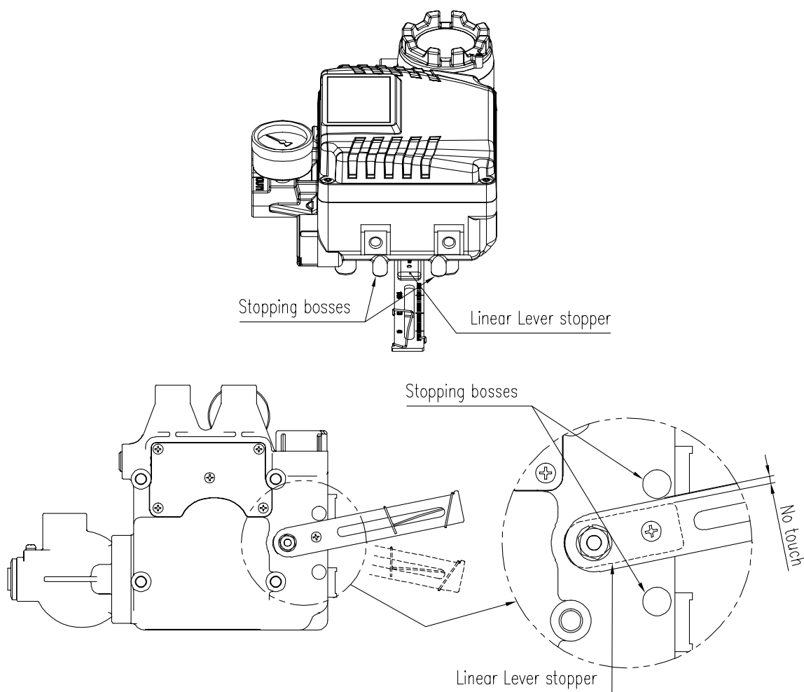
图4-9: 直行程杆止动件不得在阀门行程0 % ~ 100 %范围内触碰定位器止动凸台。
