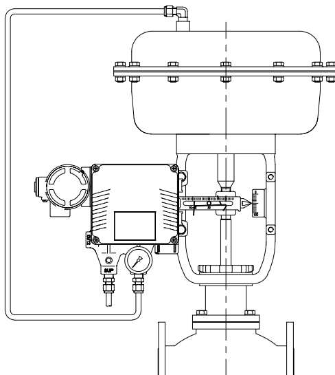
图4-2: 安装示例
