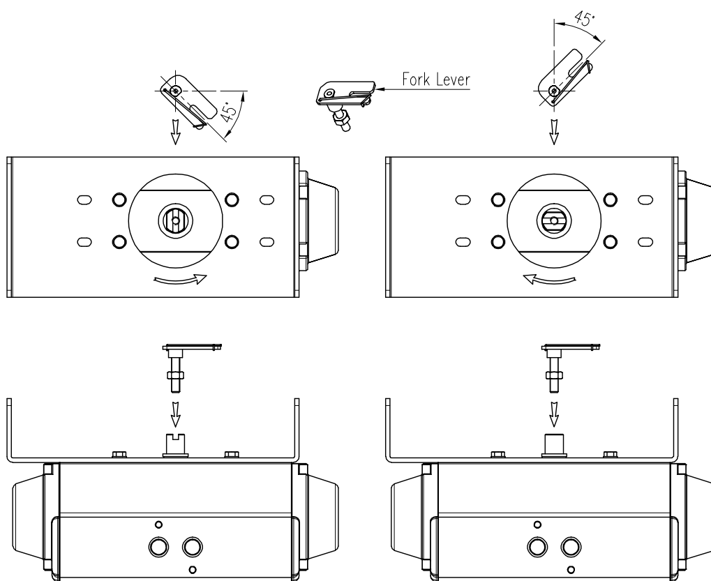
图4-15: 逆时针和顺时针方向。
