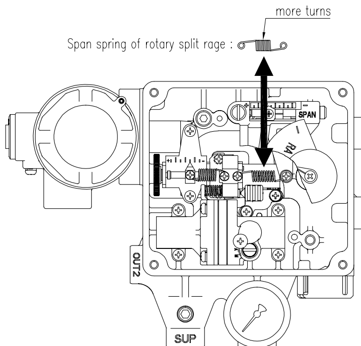
图7-18：角行程定位器
