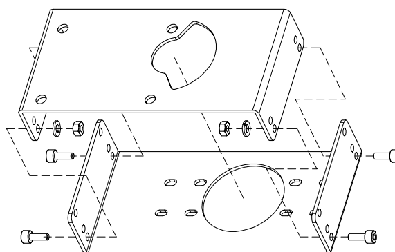
图4-14: 角行程支架组件
