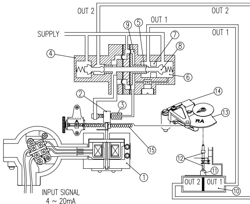
图3-2: 带执行器的角行程定位器
