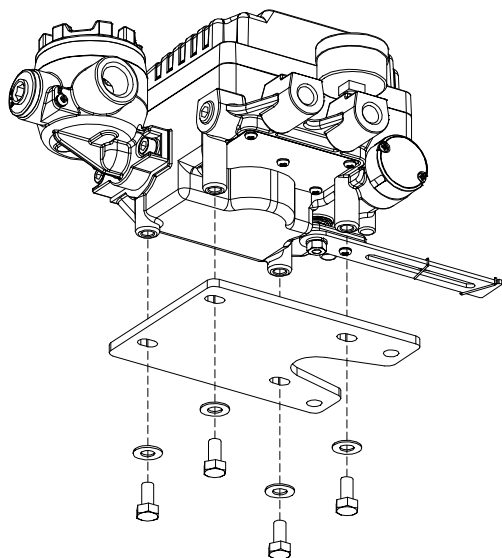
图4-3: 将定位器安装于支架上
